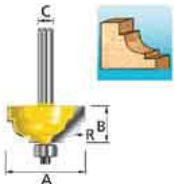
Fraises à moulurer 2 taillants à roulement G
